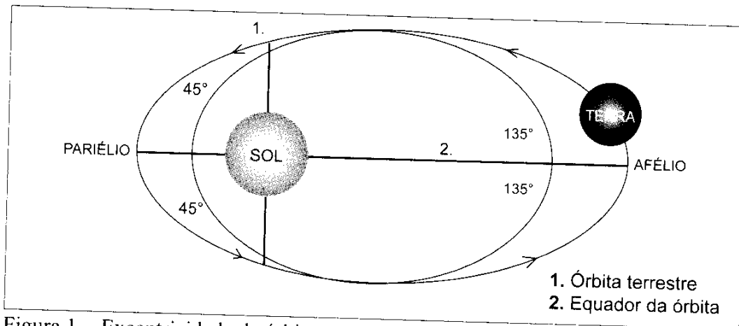
Figura 1 - Excentricidade da órbita terrestre.
