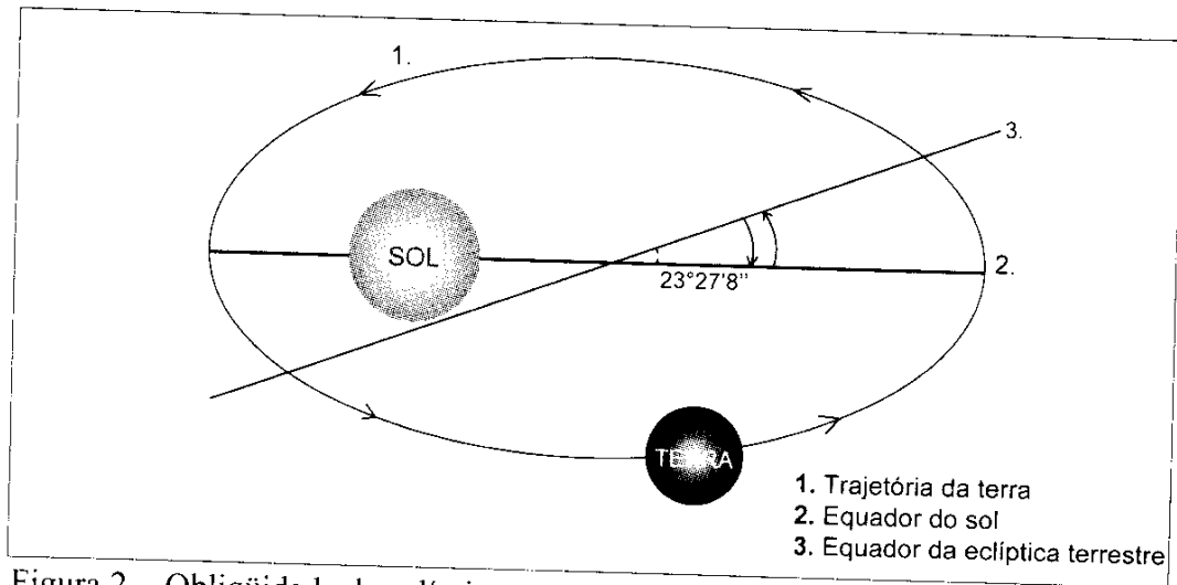
Figura 2 - Obliquidade da eclíptica terrestre terrestre.
