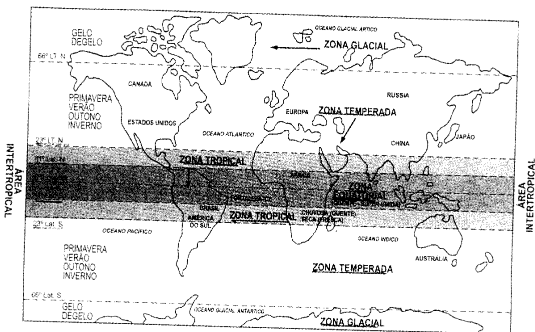
Figura 3 - Planisfério terrestre.
